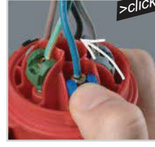
2) Terminali kapatın
