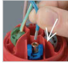
1) Kabloyu takın
