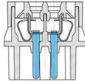
Yaylı Bağlantı
