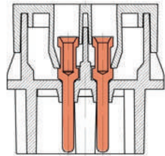
Krimp Bağlantı
