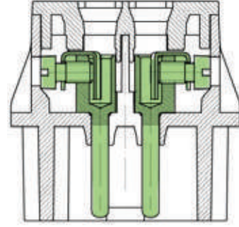
Vidalı Bağlantı
